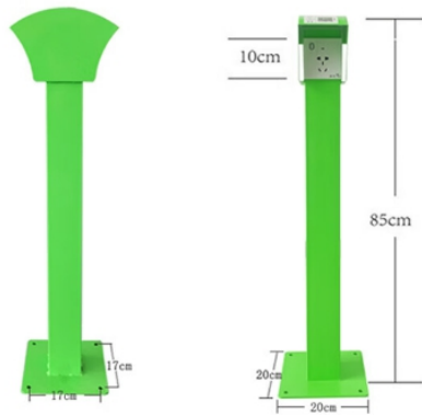
插座桩 底部孔位详情
