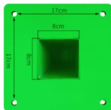
插座桩 底部孔位详情
